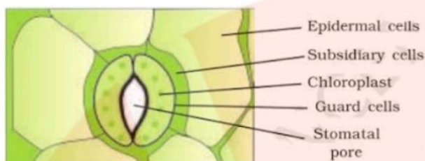
Fig.: Stomatal Apparatus
